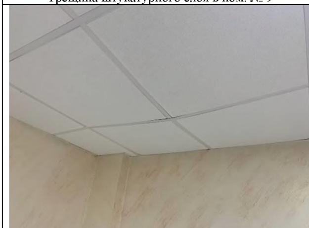
Провисание подшивного потолка в пом. № 8
